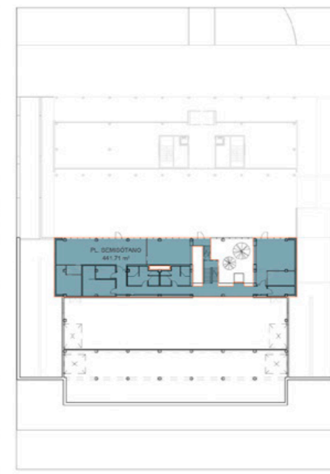
PLANTA SS
