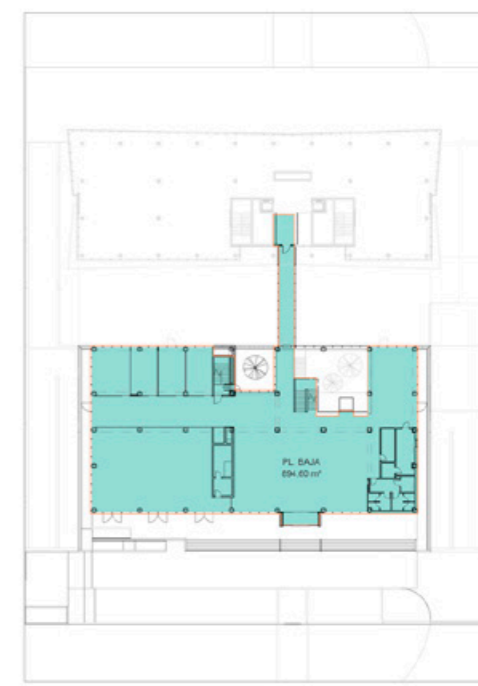
PLANTA PB
